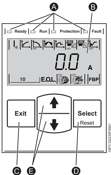
Рис. 5.1. Панель управления
