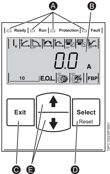
Afbeelding 5.1: HMI
