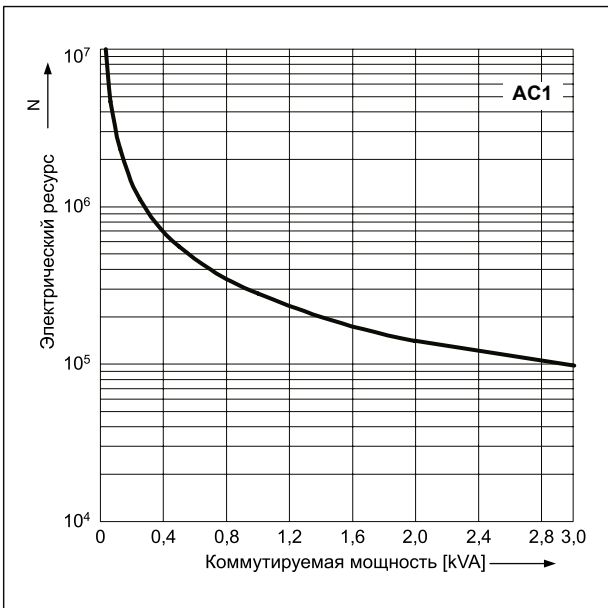
Электрический ресурс по функции мощности нагрузки. Частота коммутации: 600 циклов/час Диаг. 1
