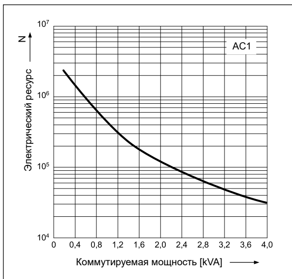
Электрический ресурс по функции мощности нагрузки. Частота коммутации: 360 циклов/час Диаг. 1
