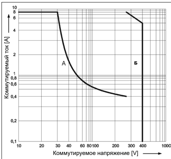
Максимальная способность коммутации A - резистивная нагрузка DC1 Б - резистивная нагрузка AC1
