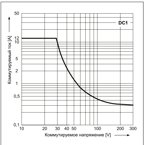
Максимальная способность коммутации для постоянного тока - резистивная нагрузка - стандартная катушка Диаг. 3
