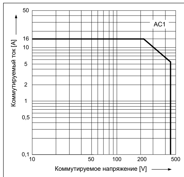
Максимальная способность коммутации для переменного тока 50 Гц - резистивная нагрузка Диаг. 2
