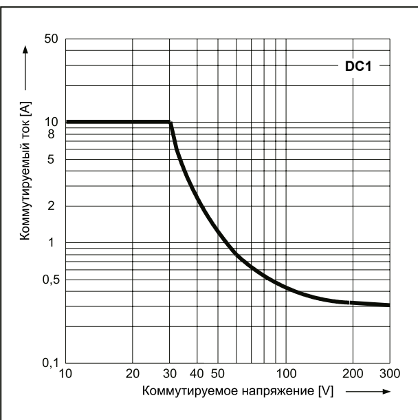
Максимальная способность коммутации для постоянного тока - резистивная нагрузка - чувствительная катушка Диаг. 4
