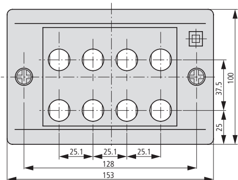
Отверстие для крепления: 2 x Ø 4,5 мм
