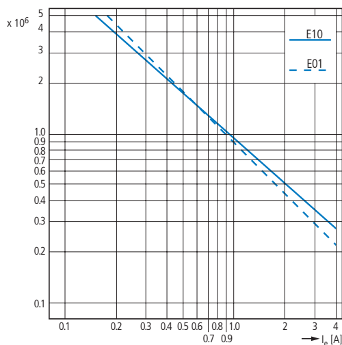
Срок службы электрических компонентов AC-15 согласно IEC/EN 60947-5-1 при 230 В I e = расчетный рабочий ток
