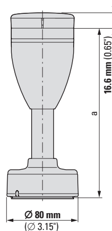
SL7-FMS-...
