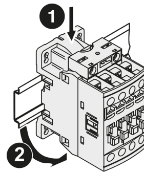
Рис. 29. Демонтаж контактора с DIN-рейки 35 мм
