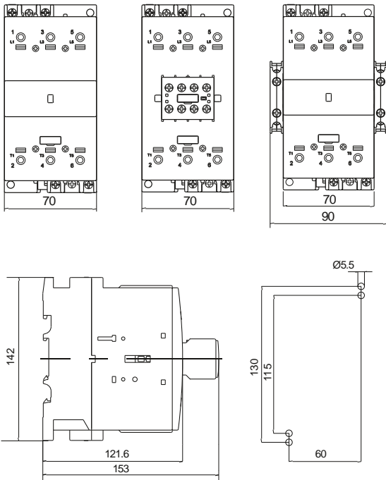
CNN 100
