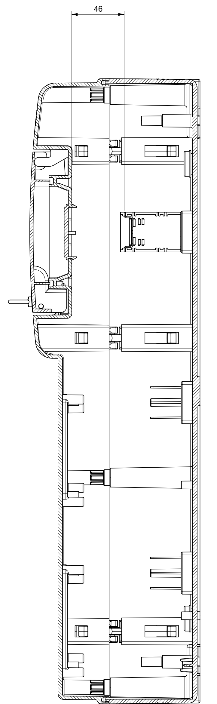
Sezione A-A
